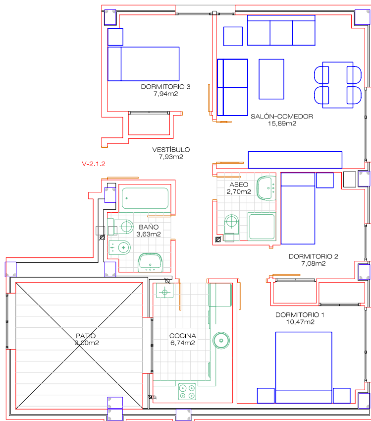
PLANO DE VIVIENDA 2.1.2 ESCALA 1/50
